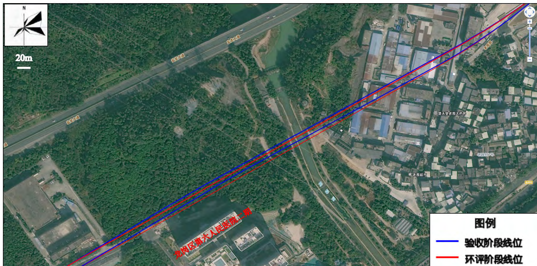
图 2.3-4 富坪站~坪地六联站线位最大位移示意图
